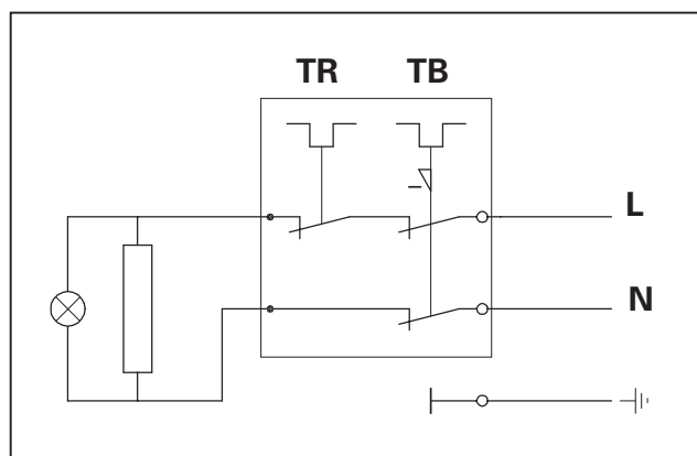
Fig. 2.3 Schéma de branchement électrique
