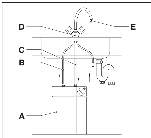
Fig. 2.2 Fonctionnement du système sans pression
