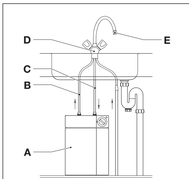
Fig. 2.2 Principewerking drukloos systeem
