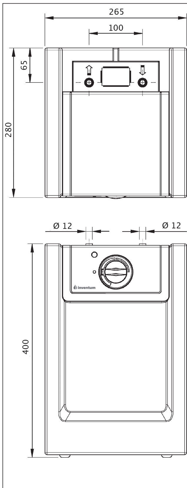
fig. 4 (Dimensions en mm)
