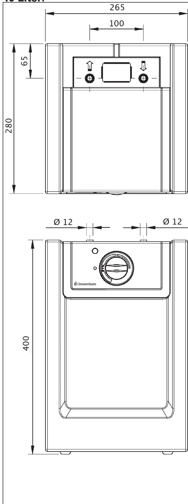
Fig. 4 (Afmetingen zijn weergegeven in mm)
