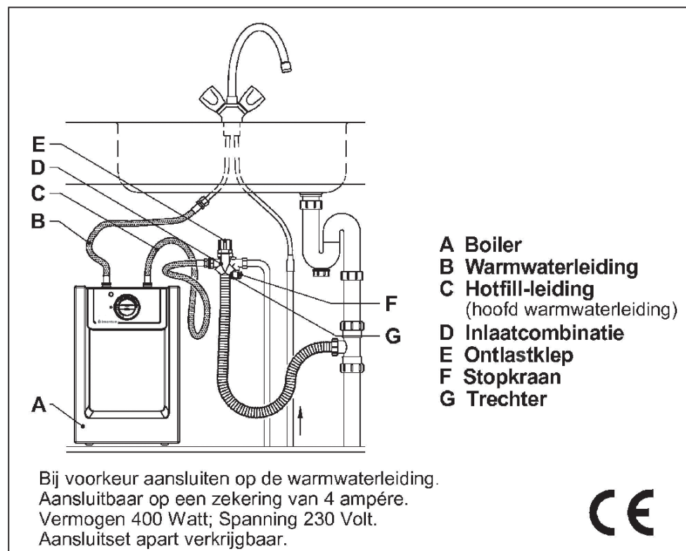
Fig. 5.2: Inventum Q10 Hotfill keukenboiler
